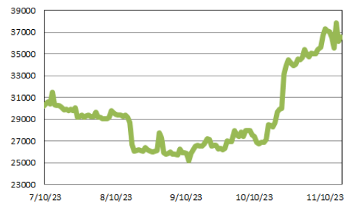
Wykres: BTC/USD
