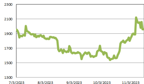
Wykres: ETH/USD
